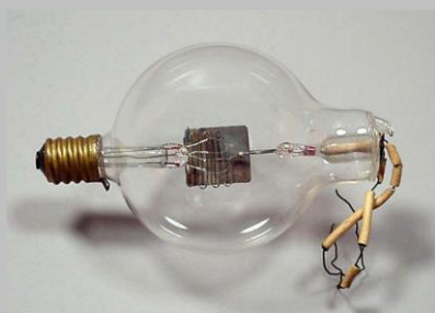
Audion esférico / Spherical Audion.
