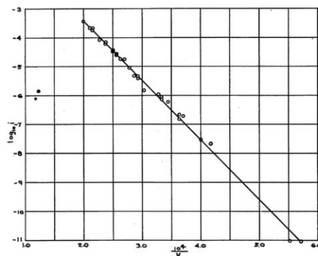
O célebre gráfico de Millikan Lauritsen
