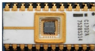
Primeira memória EPROM.
