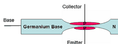
Pormenor do transístor SB100 da Philco.
