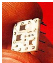
Módulo SLT da IBM para os computadores IBM 360.
