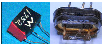
Transístor de junções crescidas num lingote de germânio.
