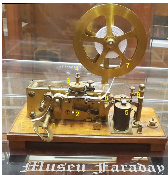
Impressor de Morse desenvolvido por Maximiliano Herrmann (1865)
