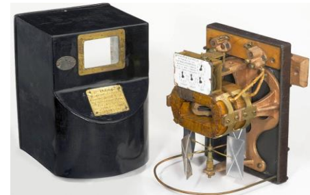
Fig. 5- Contador de Shallenberger Museu Henry Ford, EUA.
