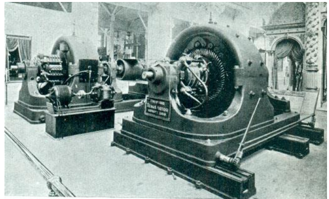
Fig.12- Alternador de 500 hp na expo de 1893.
