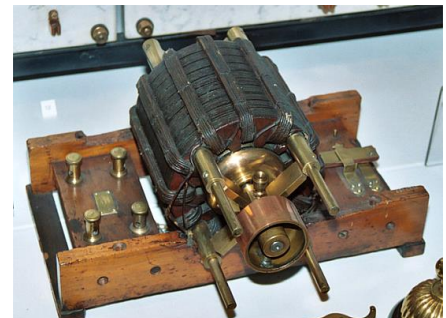
Fig. 4- Motor de indução de 1877 – 1878 Museu Britânico de Ciências, em Londres.
