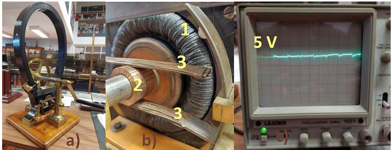
Fig 3 - Dínamo de Gramme/Breguet nº 100 (Museu Faraday). a) -aspecto geral, b) - detalhe do induzido e c) - tensão gerada.
