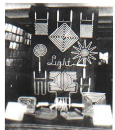
Fig.15- Exemplo de lâmpadas “Wireless” apresentadas em 1893 na sala escura.
